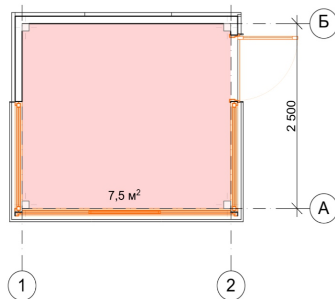
План на отметке 0,000 М 1:50
