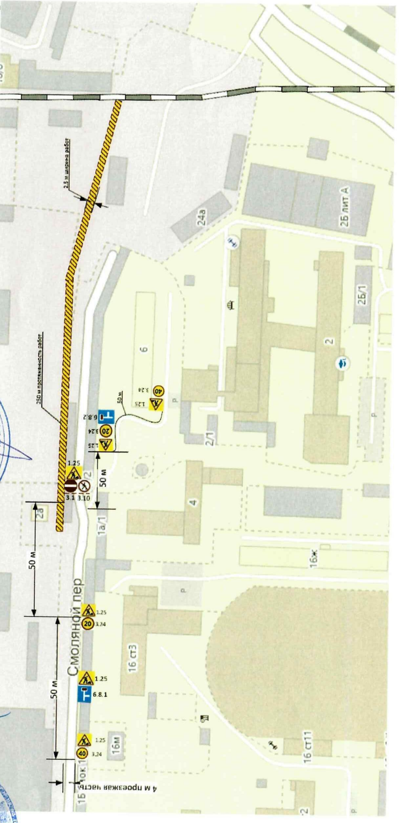
Схема расположения технических средств организации дорожного движения на время проведения ремонтных работ.
