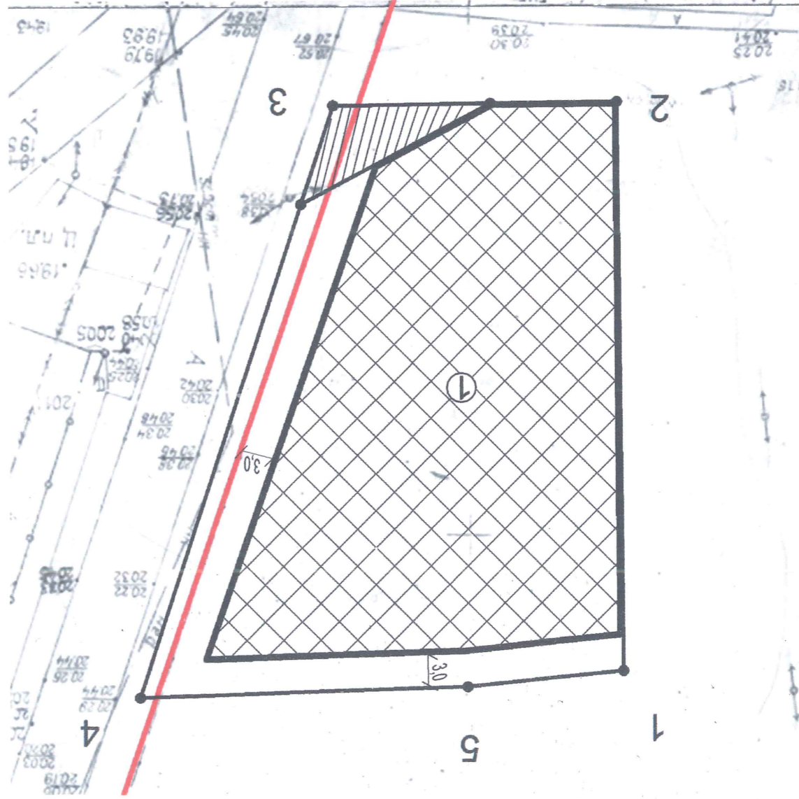
Чертеж градостроительного плана земельного участка и линий регулирования
